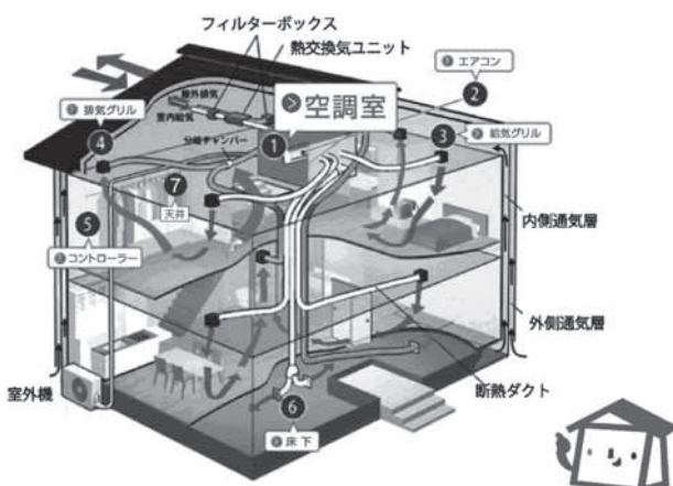
マッハシステムの仕組み
